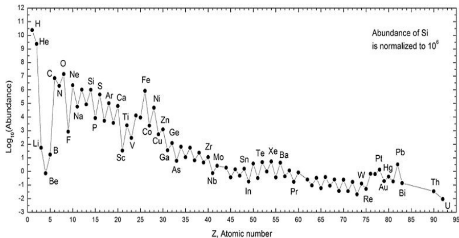
太阳系前 92 种化学元素的丰度
